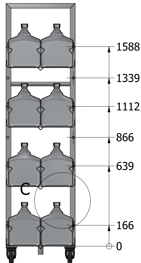
A-A ( 1 : 18 )
