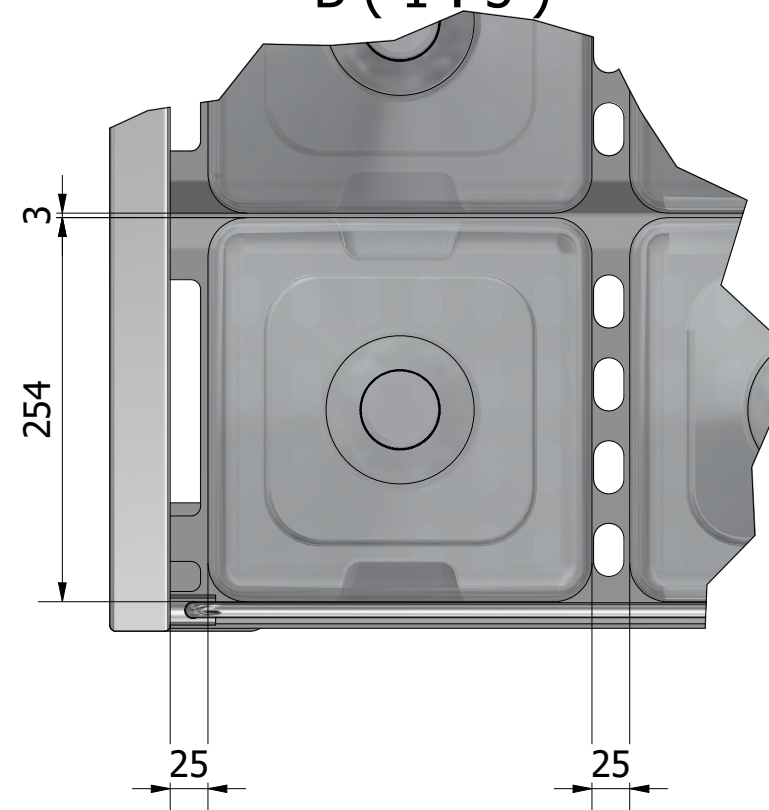
B ( 1 : 5 )
