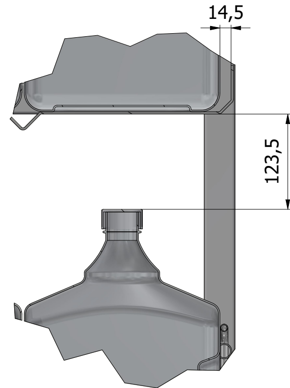
C ( 1 : 5 )
